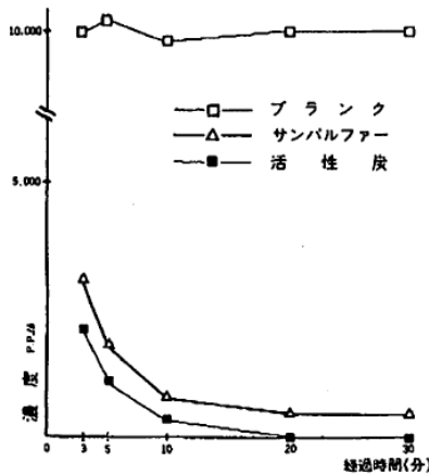
ガス吸着性能表 アンモニア
