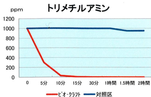
トリメチルアミン 魚の腐ったようなニオイ
