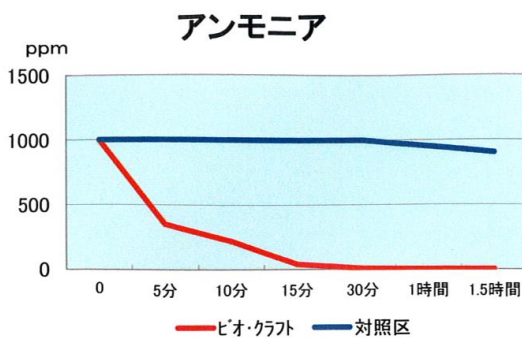
アンモニア 畜尿中の窒素化合物が分解したときに発生する
